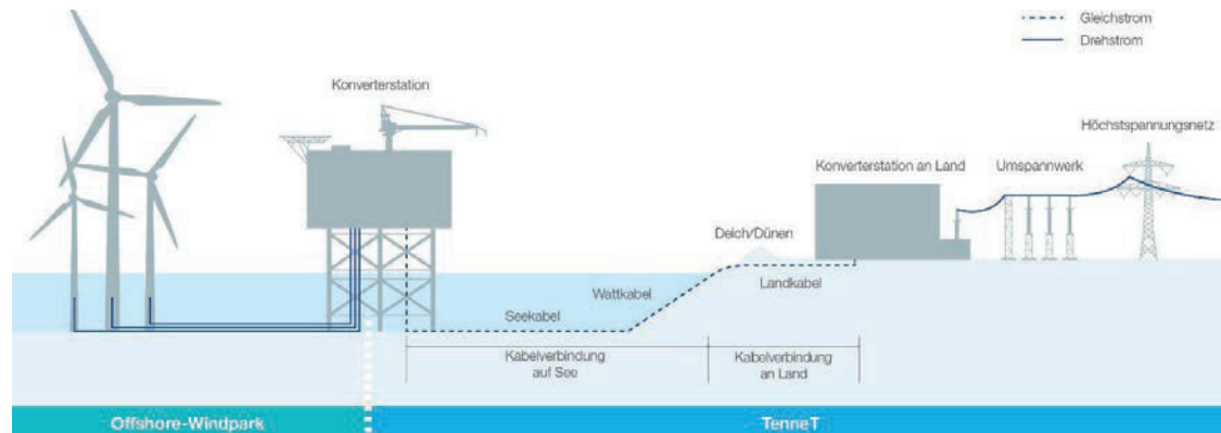
Mit dem innovativen 66-kV-Anschluss werden die Windparks direkt mit der Offshore-Plattform von TenneT verbunden. © TenneT
